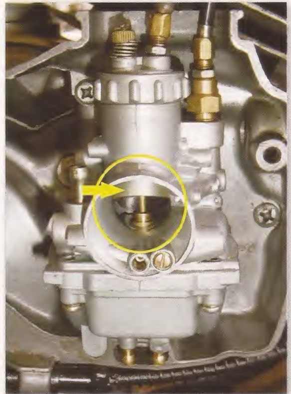
Carburador de venturi variable
